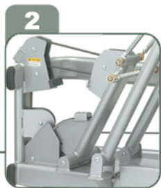
地平線的中心軸與長度不一的四連桿結構 Floor Level Pivot and Unequal Length Four-bar Linkage
